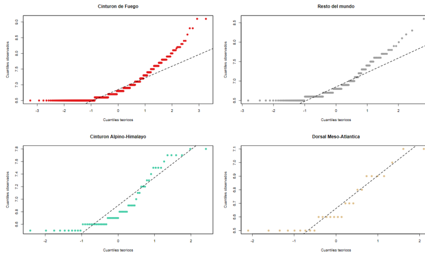
Figura 1. QQ-plots de magnitud por zona sísmica.
