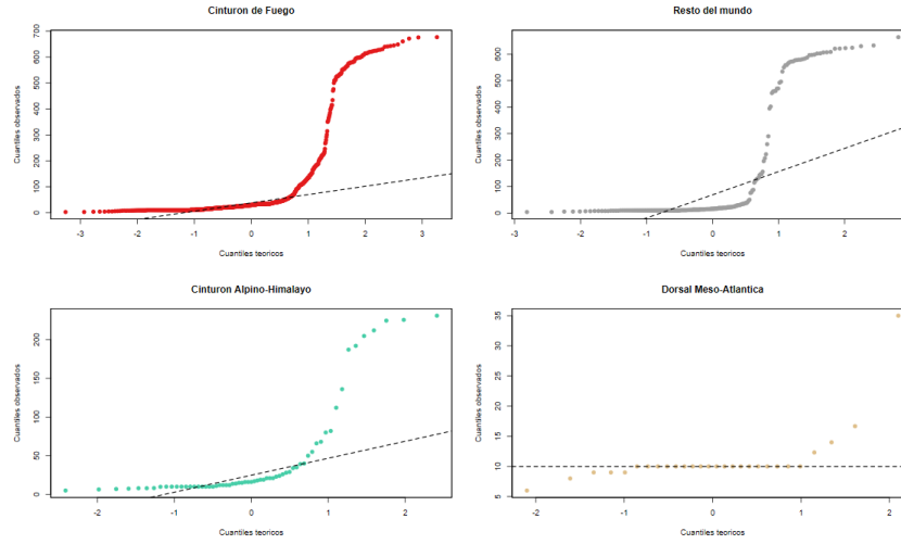
Figura 2. QQ-plots de profundidad por zona sísmica.
