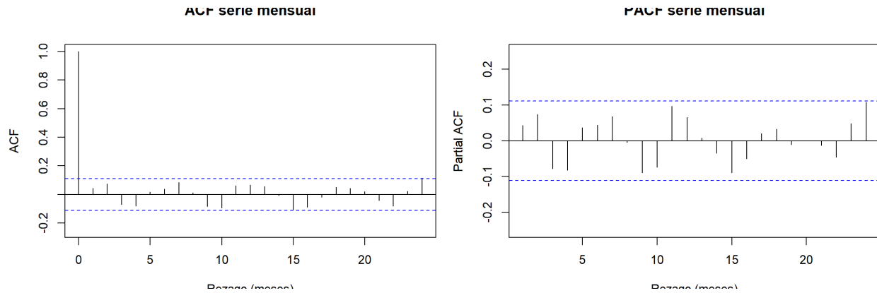
Figura 5. ACF y PACF de la serie mensual de conteos del catálogo.
