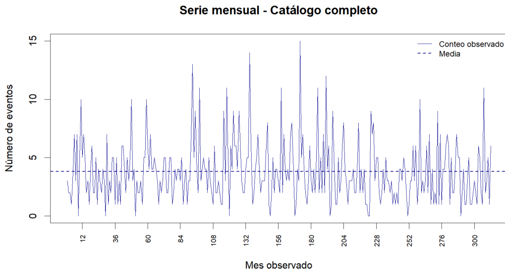
Figura 4. Serie mensual de eventos del catálogo completo.
